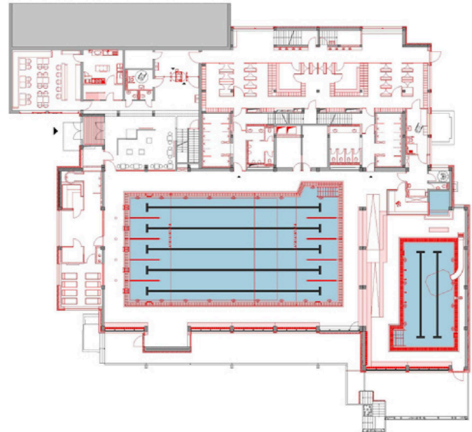
Grundriss Erdgeschoss
