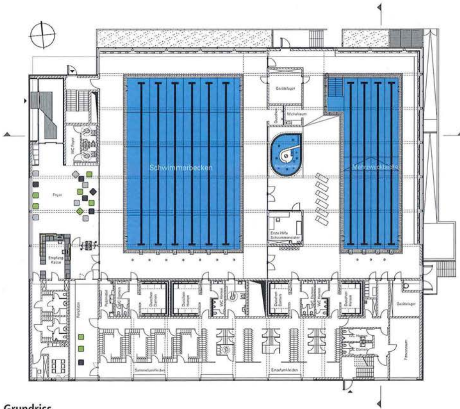
Grundriss
